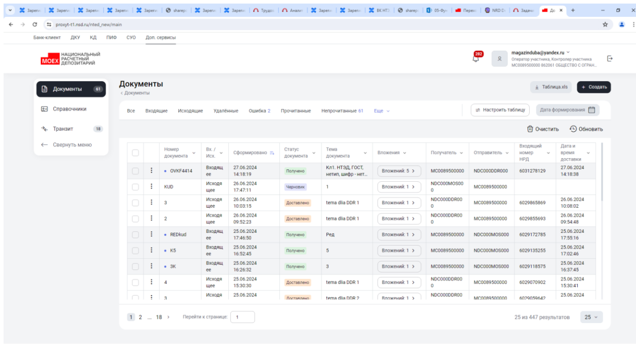
Рисунок 3 Главная страница
