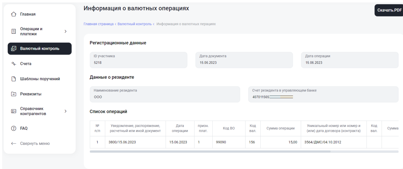
Рисунок 6.3. ИВО
