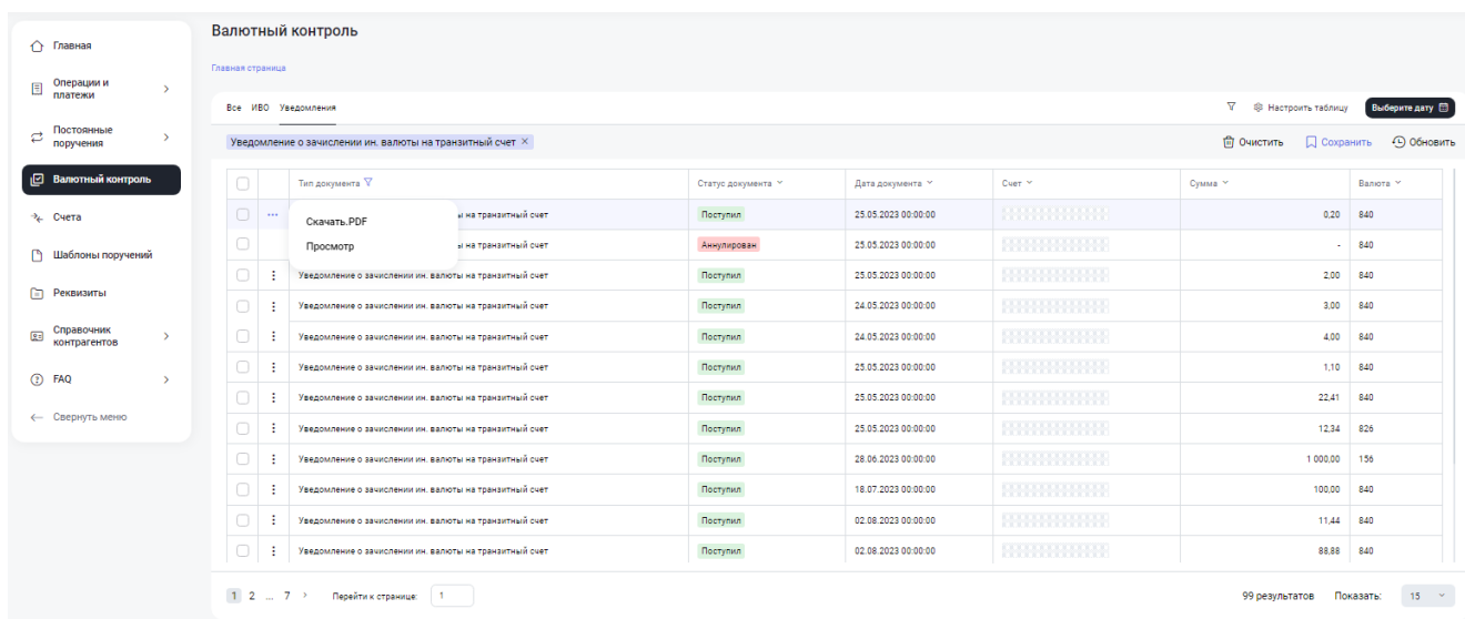
Рисунок 6.4. Просмотр Уведомления
